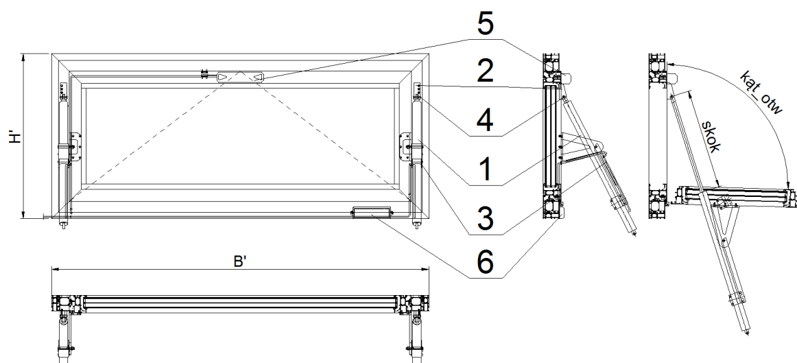
1 – siłowniki wrzecionowe, 2 – uchwyt górny, 3 – uchwyt dolny z zaczepem i obejmą przesunięcia punktu obrotu, 4 – trzpień górny, 5 – elektroygiel obrotowy, 6 – interfejs rygla
